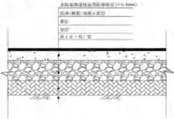
图 4-6 生产区地坪防渗结构示意图
