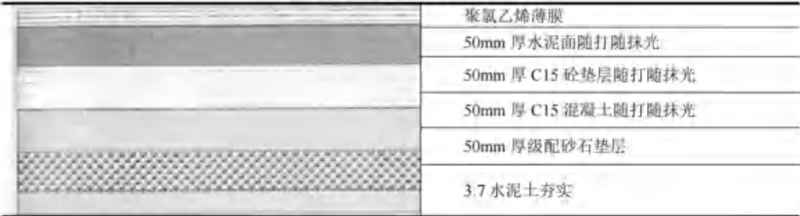
图 4-7 危废仓库防渗结构示意图
