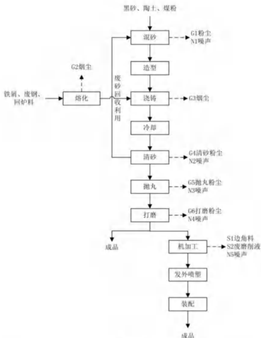
图 2-5 原项目生产工艺流程图 (Gn 废气; Sn 固体废弃物; N 噪声)
