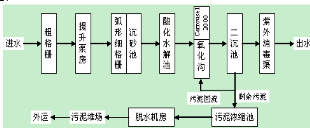
图 4-2 武南污水处理厂废水处理工艺流程
