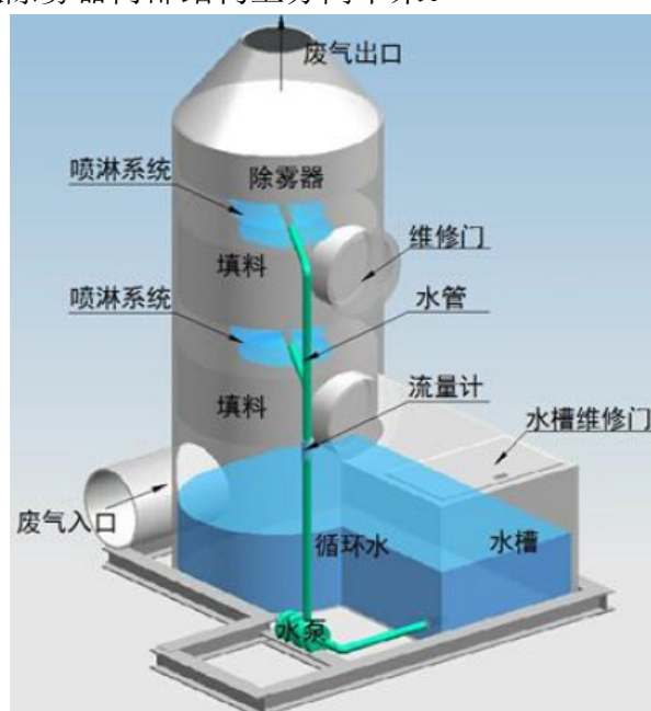
图 4-2（2） 喷淋塔示意图
