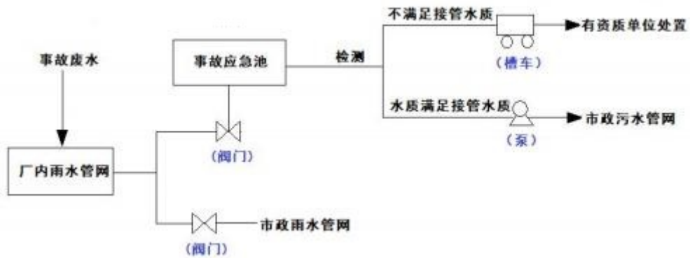
图 4-4 事故排水控制和封堵示意图
