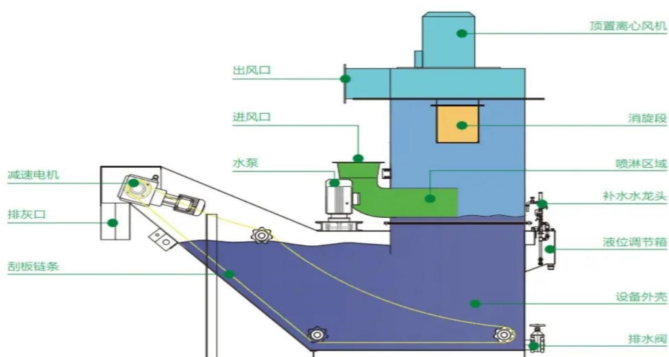
图 4-2（1） 湿式除尘一体机（文丘里）示意图
