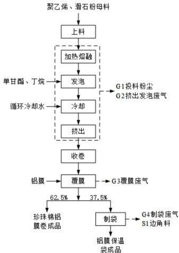
图 2-3 工艺流程图
