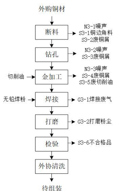
图 2-3 铜件生产工艺流程图
