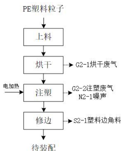
图 2-3 塑料制品生产工艺流程图
