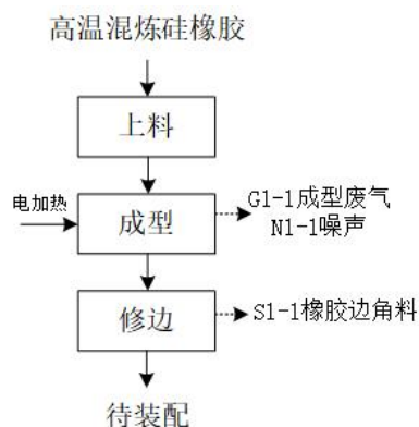
图 2-2 橡胶制品生产工艺流程图
