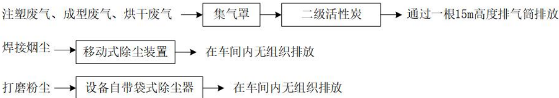
图 4-1 废气处理工艺示意图
