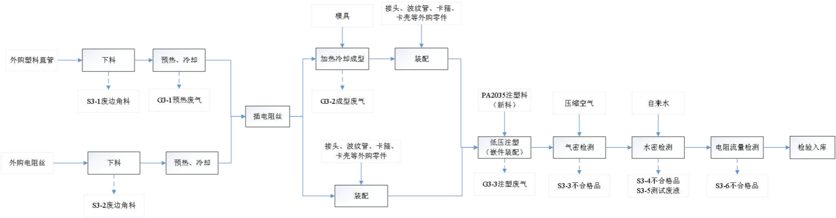
图 2-4 UTS 流体管路系统-塑料管工艺流程图
