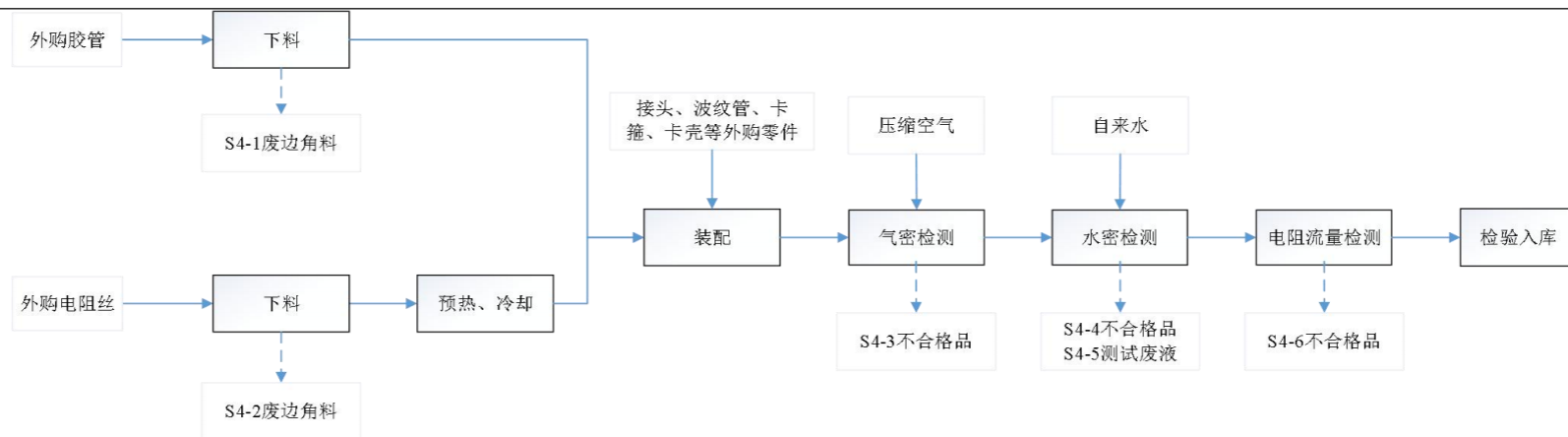
图 2-5 UTS 流体管路系统-胶管工艺流程图
