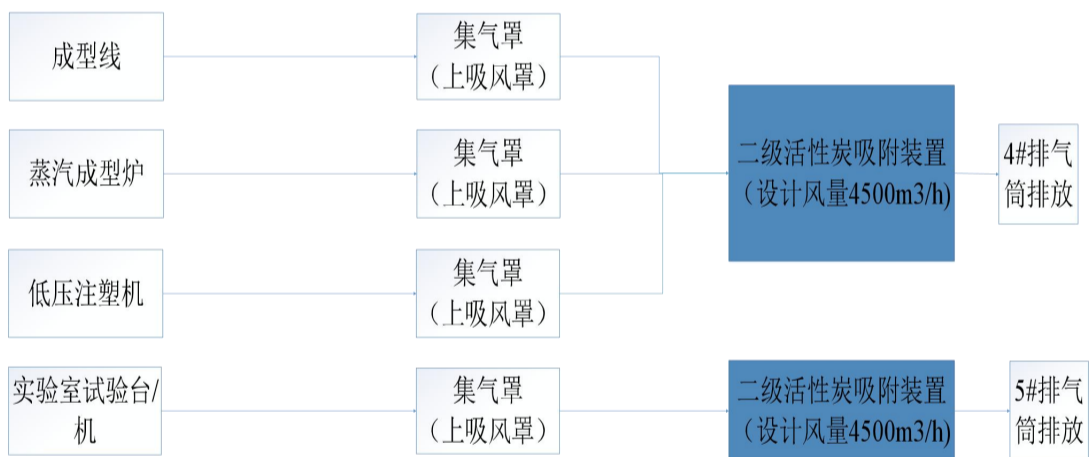
图 4-1 本项目废气处理流程图
