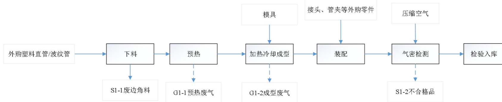
图 2-2 普通流体管路系统-塑料直管、波纹管生产工艺流程图
