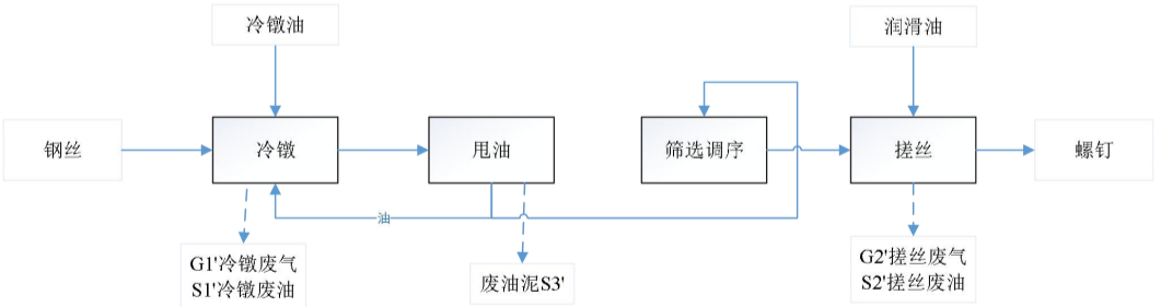
图 2-7 螺钉生产工艺流程图
