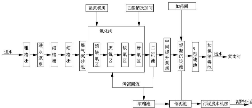
图 4-4 武南第二污水处理厂处理工艺流程图
