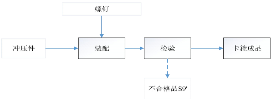
图 2-9 卡箍生产工艺流程图
