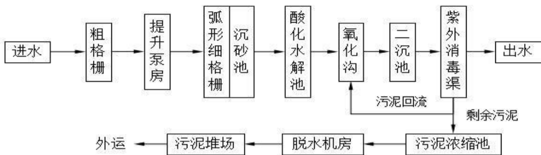
图 4-3 武南污水处理厂处理工艺流程图
