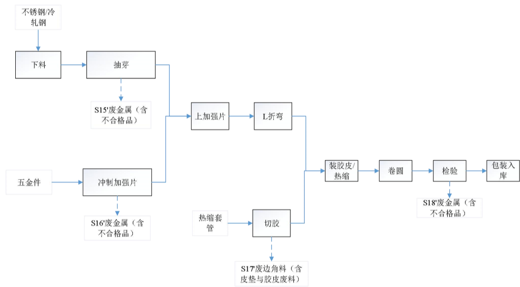
图 2-11 线卡生产流程图
