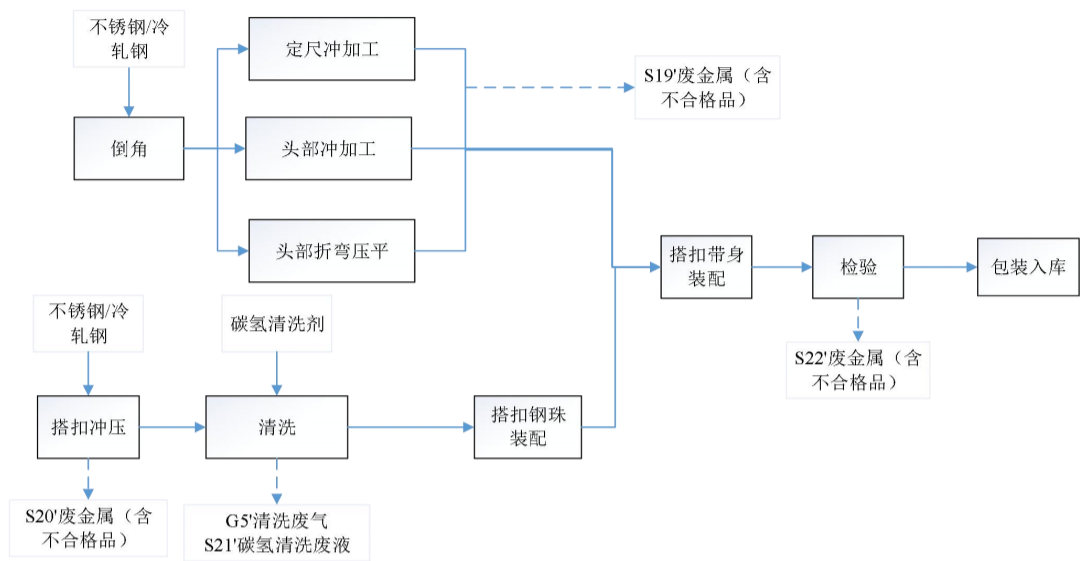
图 2-12 扎带生产流程图
