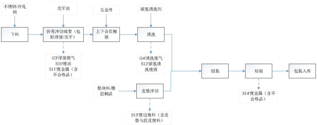
图 2-10 电缆夹箍生产流程图
