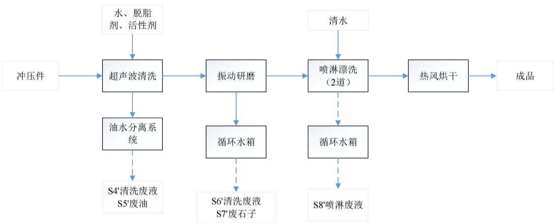
图 2-8 冲压件去毛刺清洗工艺流程图
