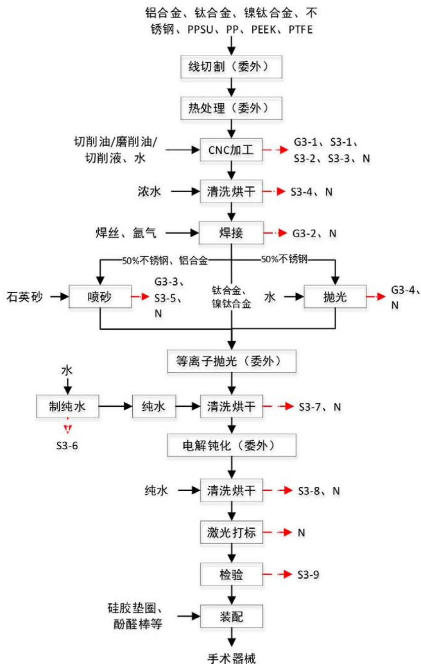
图 2-4 手术器械生产工艺流程图
