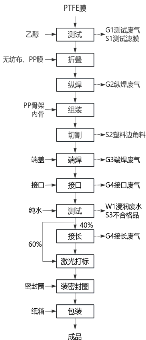
图 2-2 工艺流程图
