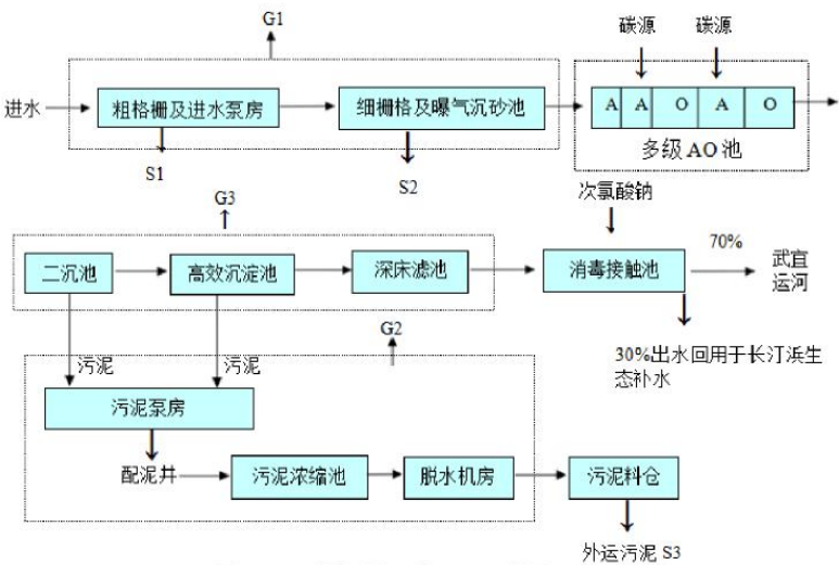
图 4-4 滨湖污水处理厂工艺流程图
