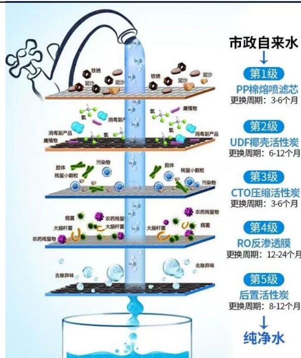
图 2-2 纯水制备工艺流程图
