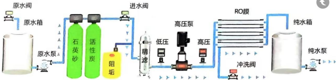
图 4-3 厂内废水处理设施工艺流程图
