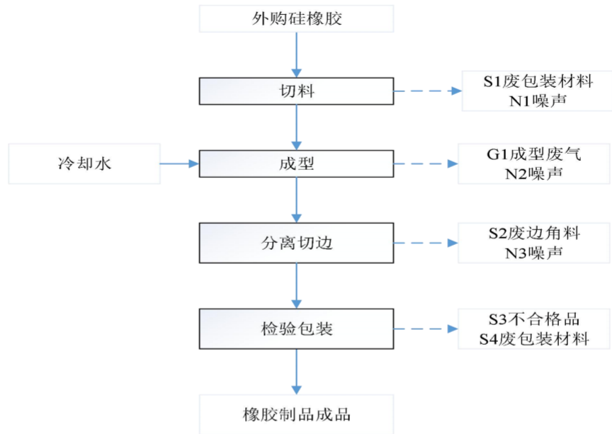
图 2-2 橡胶制品工艺流程图
