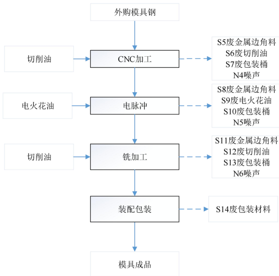
图 2-2 橡胶模具工艺流程图
