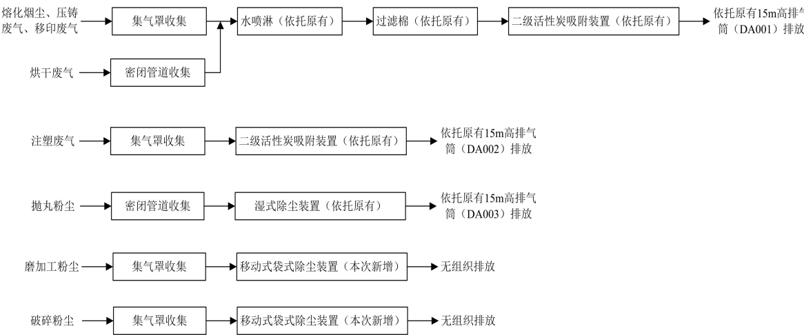
图 4-1 废气收集及处理工艺示意图
