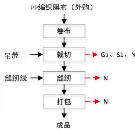
图 2-3 集装袋生产工艺流程图 (注：Gn：废气污染物；Sn：固体废弃物；N：噪声)
