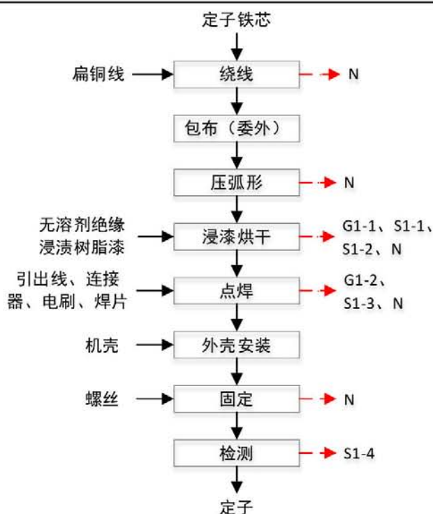
图 2-2 定子生产工艺流程图 (注: Gn: 废气污染物; Sn: 固体废弃物; N: 噪声)
