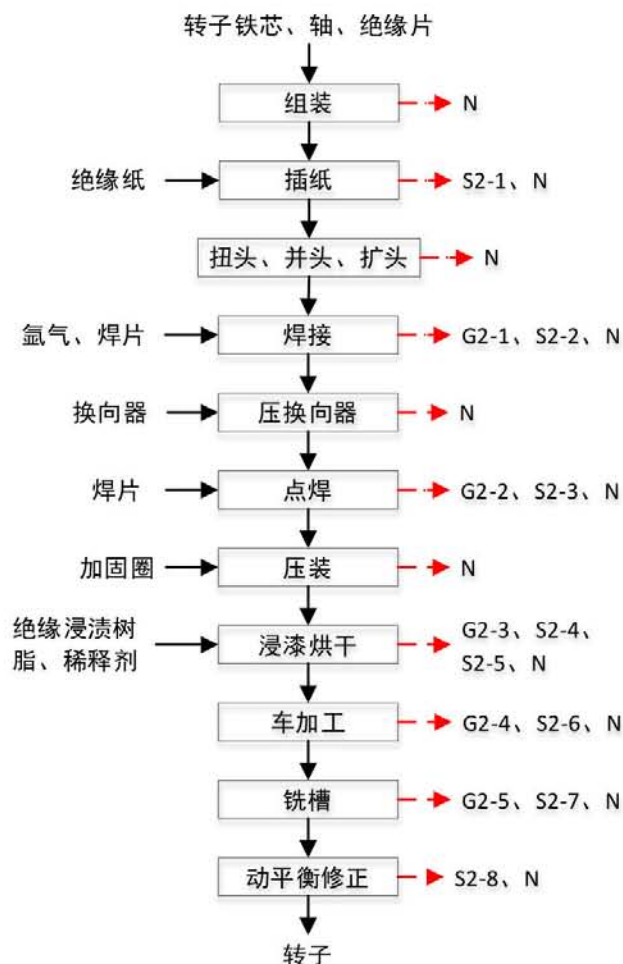
图 2-3 转子生产工艺流程图
