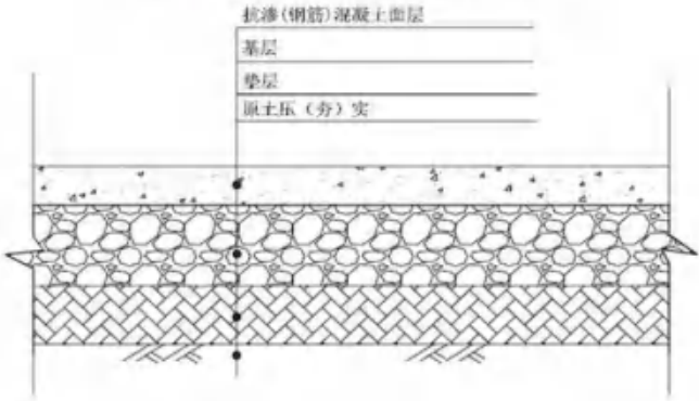
图 4-7 一般污染防治区典型防渗结构示意图
