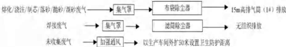
图 4-1 废气处理流程图
