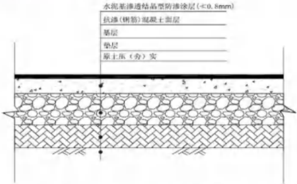
图 4-5 生产区地坪防渗结构示意图
