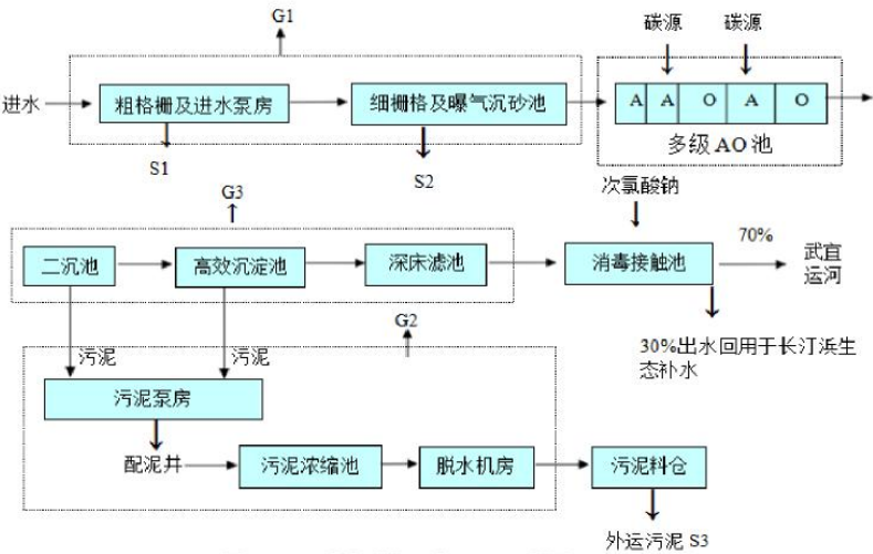
图 4-4 滨湖污水处理厂工艺流程图
