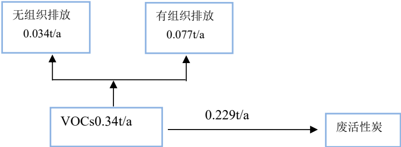
图 2-1 本项目 VOCs 平衡图
