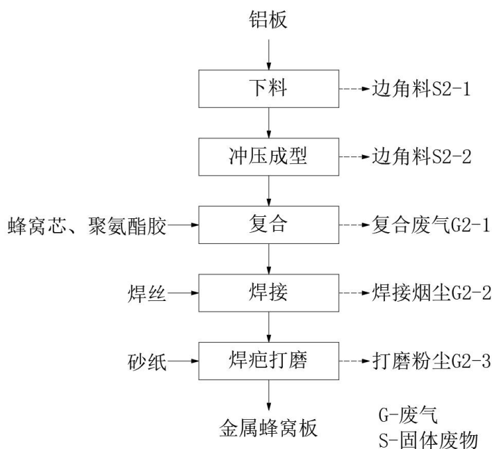
图 2.2-2 金属蜂窝板制造工艺流程及产污环节图
