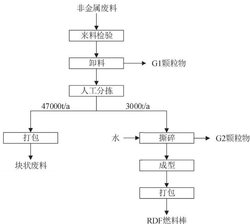
图 1 本项目工艺流程图
