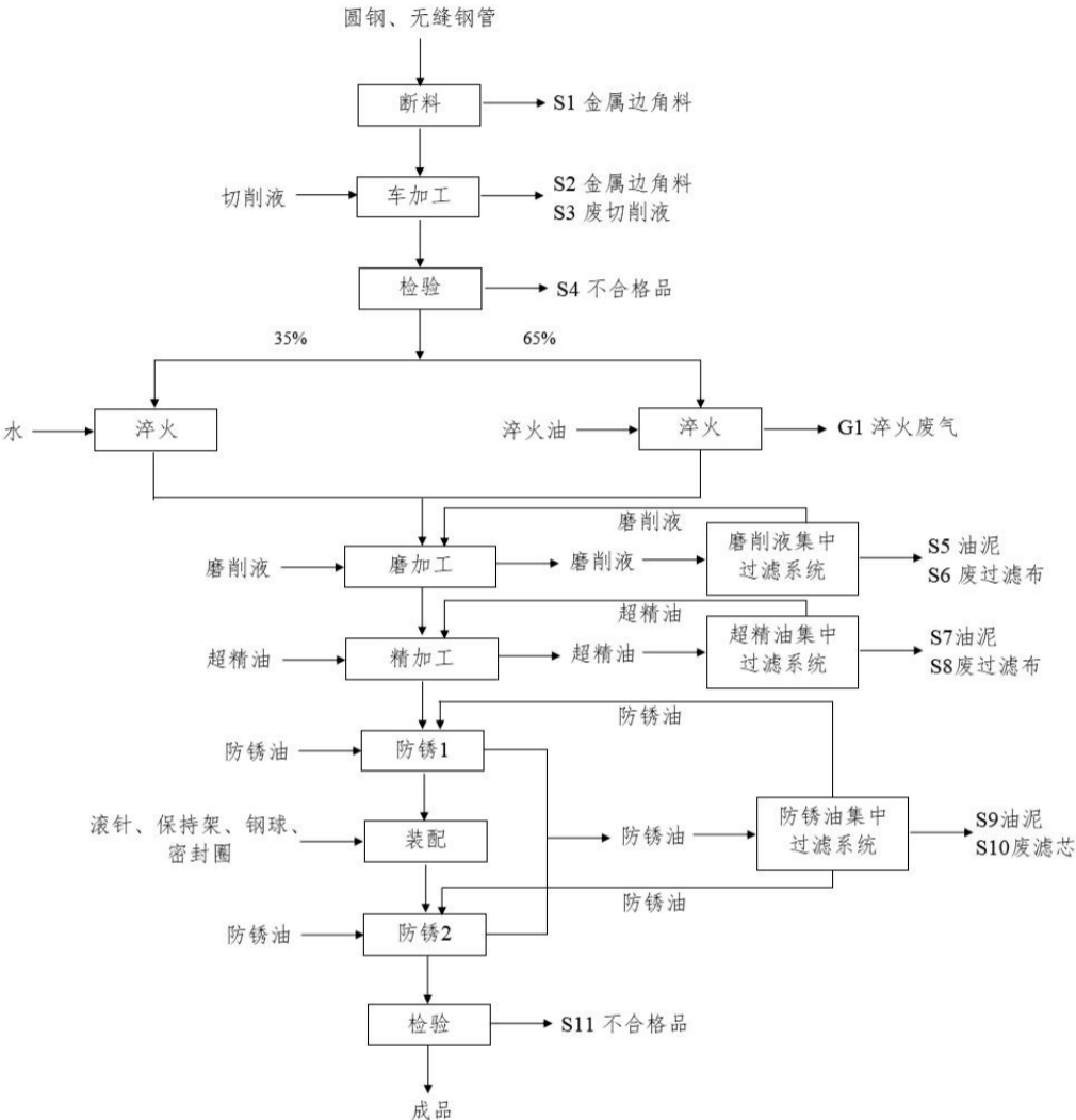
图2-5 轴承生产工艺流程图
