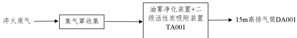
图 4-1 本项目废气处理流程图
