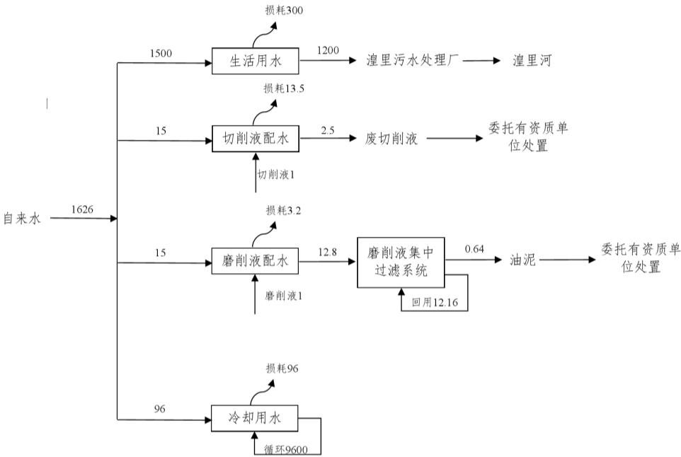
图 2-2 本项目水平衡图 单位 m³/a
