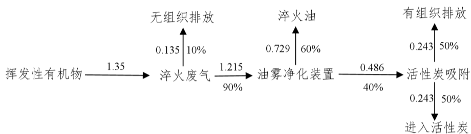
图 2-4 挥发性有机物平衡图 单位 t/a
