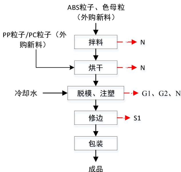
图 2-2 塑料制品生产工艺流程图
