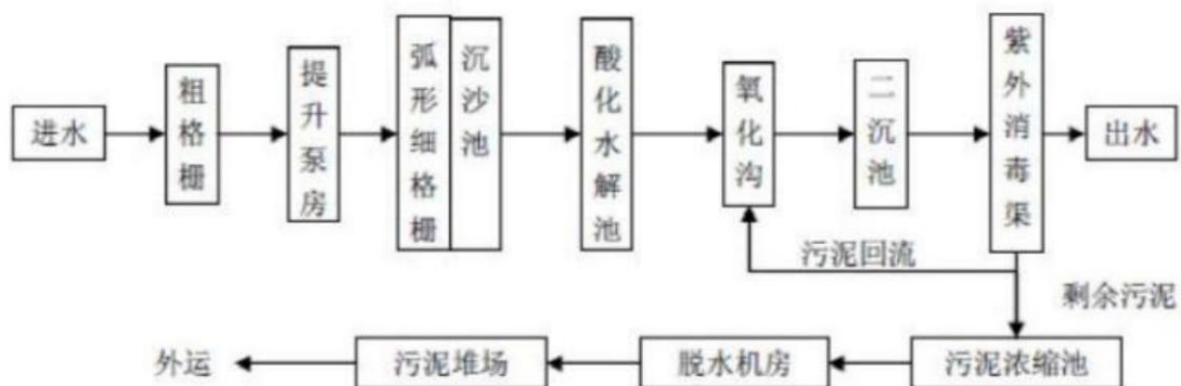
图 4.1-1 武南污水处理厂污水处理工艺流程图
