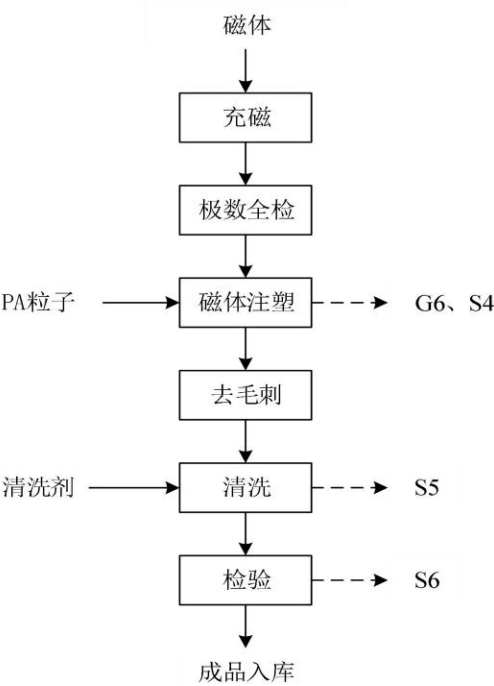
图 2.2-2 磁体组件生产工艺流程图
