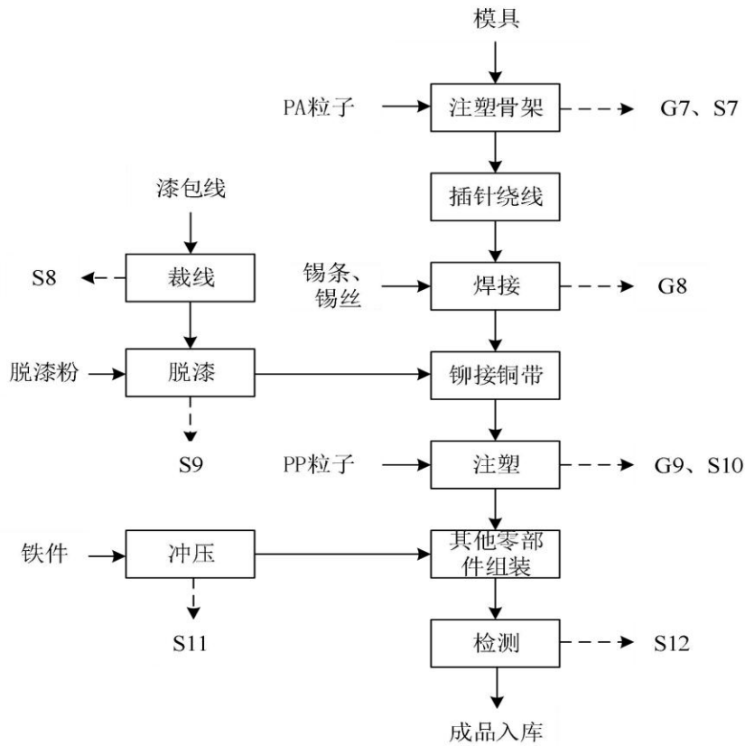
图2.2-3 测速器生产工艺流程图
