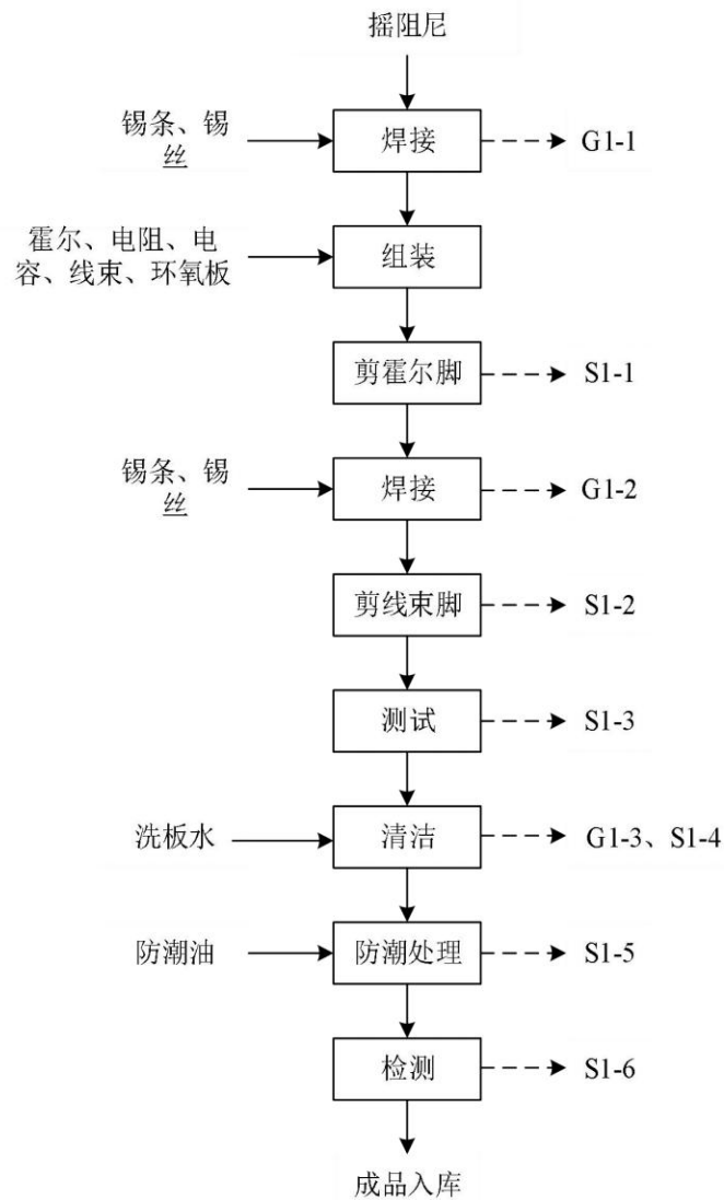
图 2.3-1 PG 霍尔板生产工艺流程图
