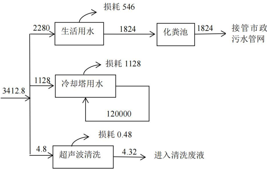
图 2.1-1 本项目水平衡图 单位：t/a
