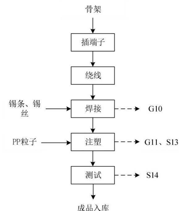
图 2.2-4 空气悬挂、电子线圈生产工艺流程图
