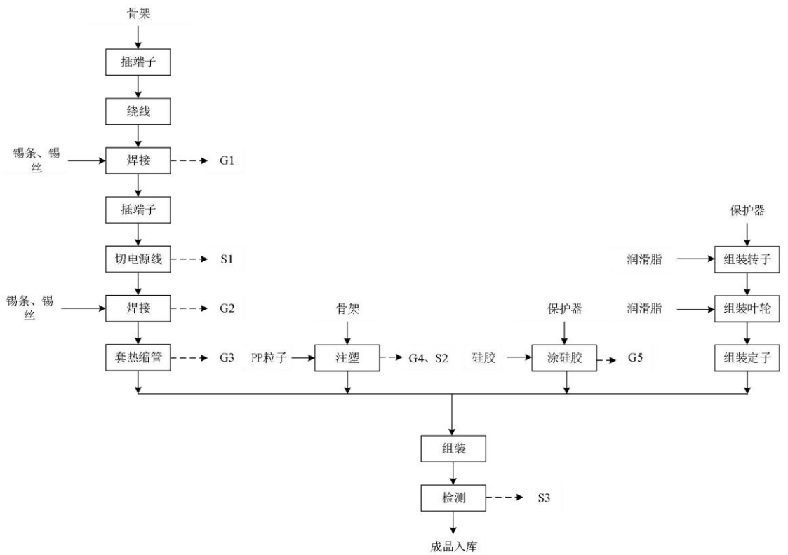
图 2.2-1 本项目排水泵生产工艺流程及产污环节图
