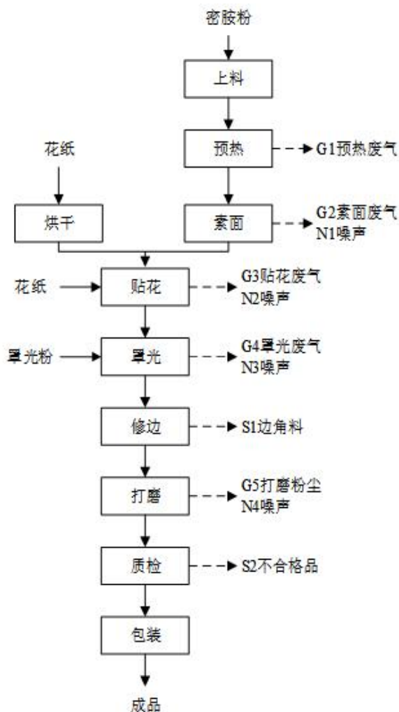
图 2-2 密胺餐具生产流程图
