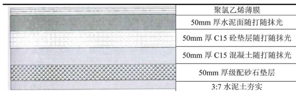
图4-3 危废仓库防渗结构示意图
