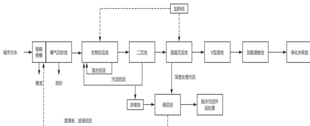
图4-1 武南污水处理厂工艺流程图
