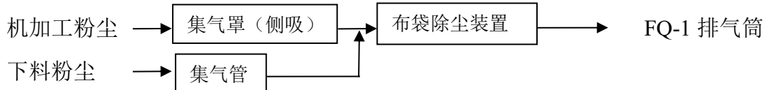
图 4-1 本项目废气管线图
