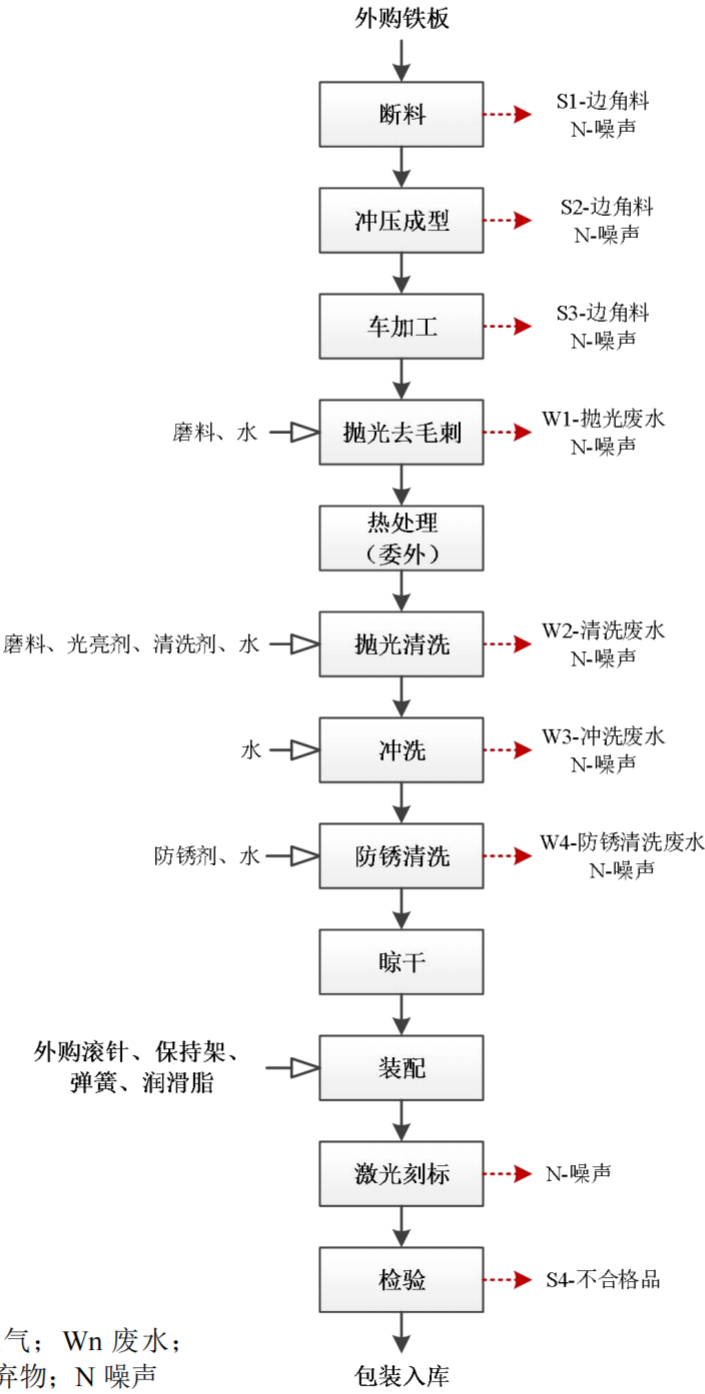
图 2-2 新能源汽车零部件生产工艺流程图
