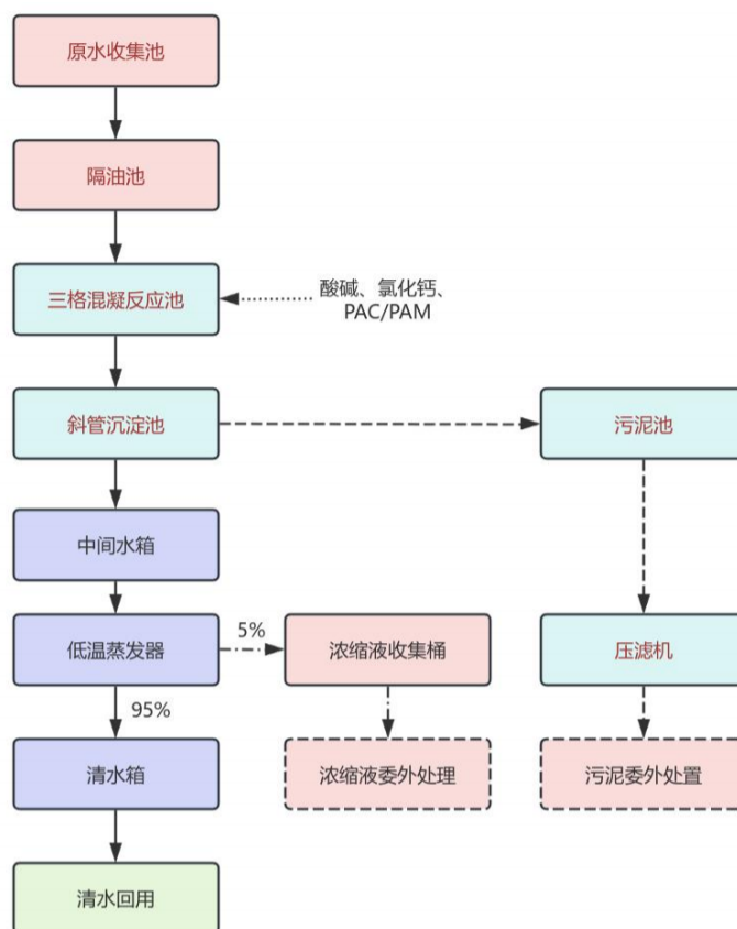
图 4-1 工业废水处理流程图
