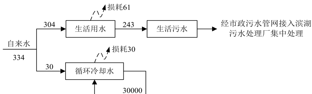
图 2-1 企业水平衡图（单位：t/a）
