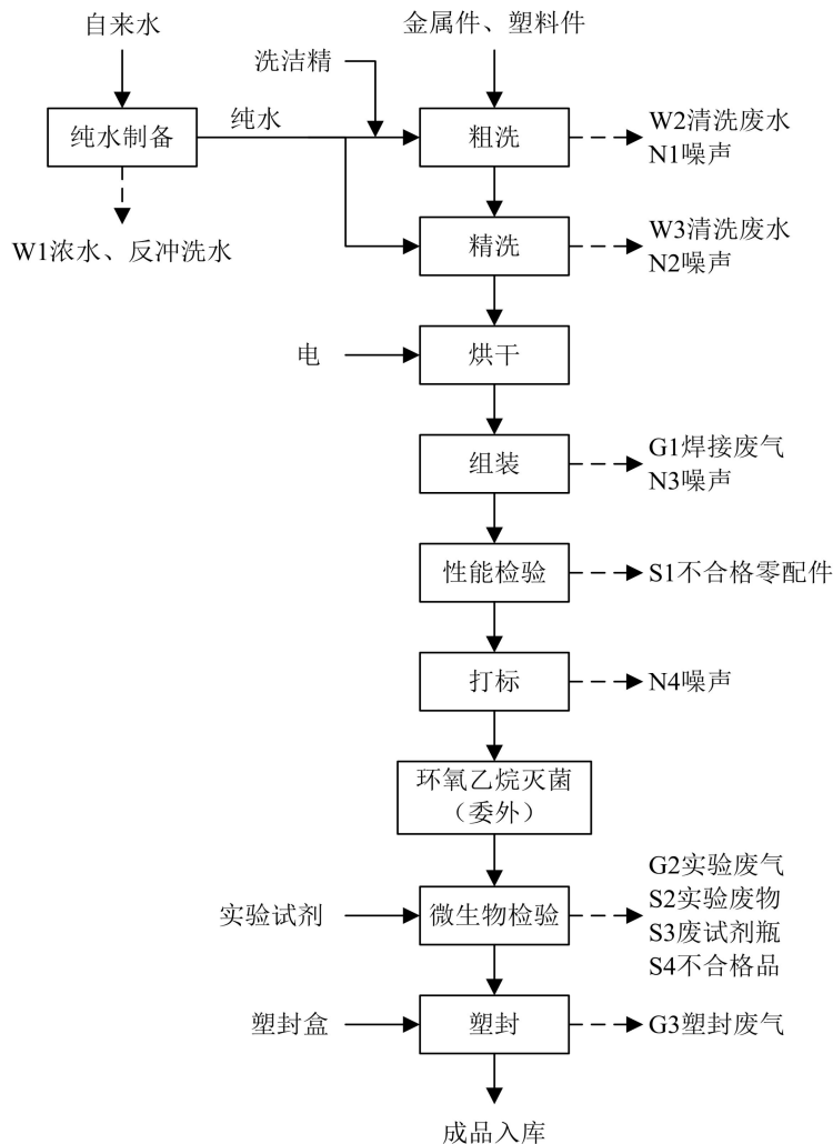
图 2-2 生产工艺流程图
