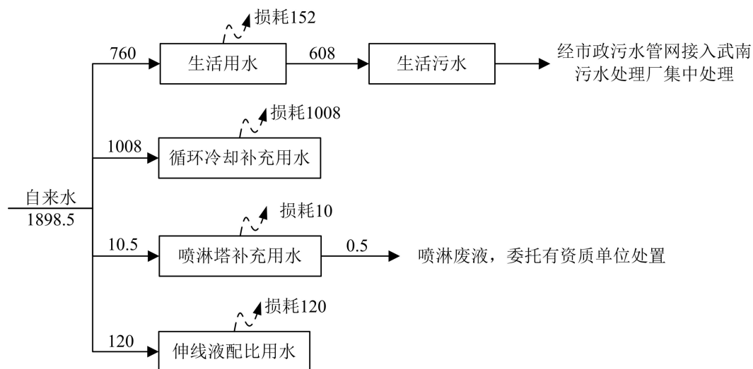
图 2-1 企业水平衡图（单位：t/a）
