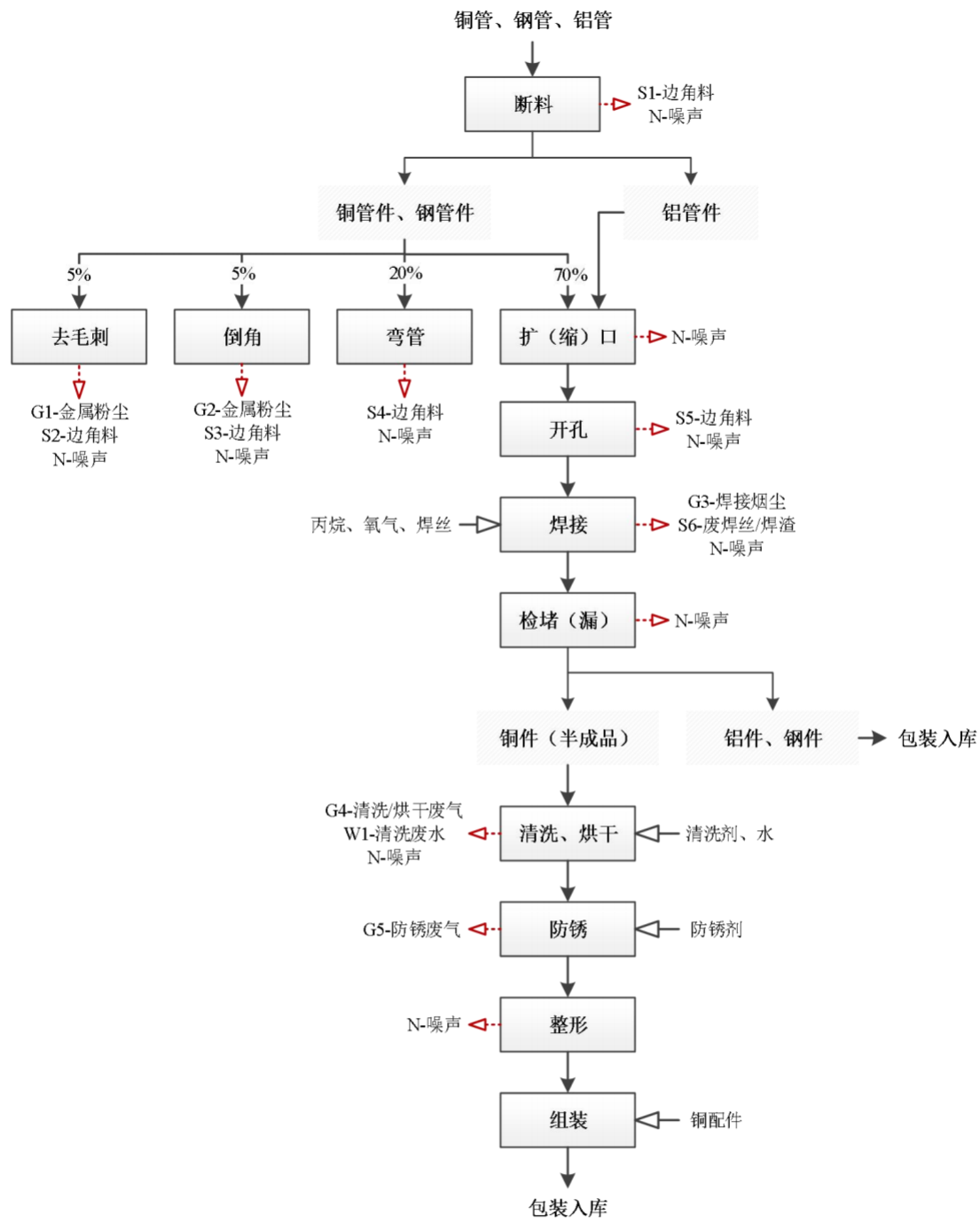
图 2-2 制冷设备配件生产工艺流程图
