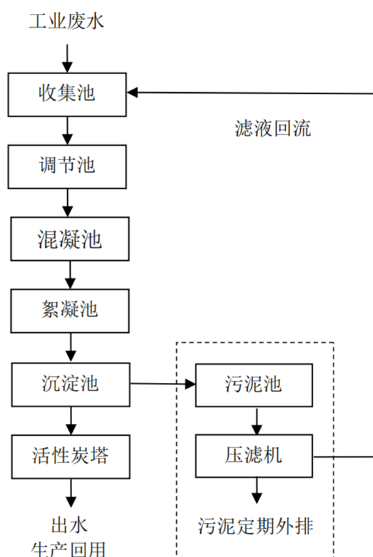
图4-3工业废水处理流程图
