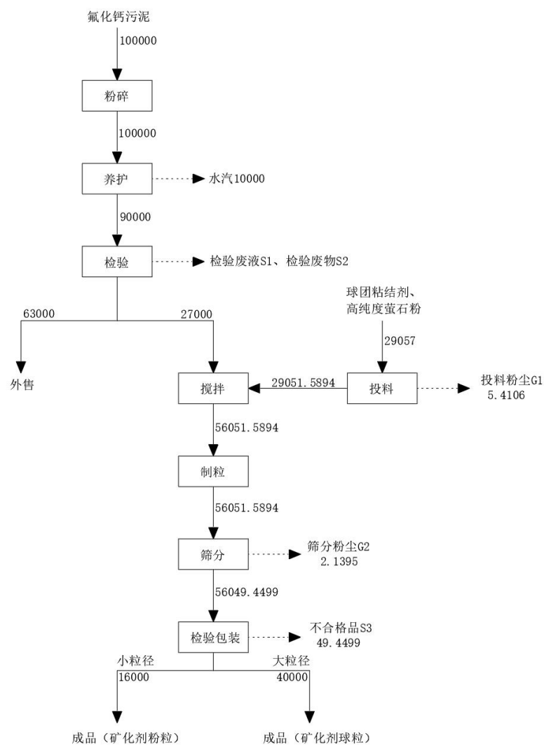
图 2-3 矿化剂生产物料平衡图 (t/a)
