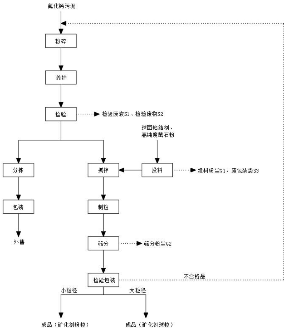
图 2-4 氟化钙污泥工艺及产污流程图
