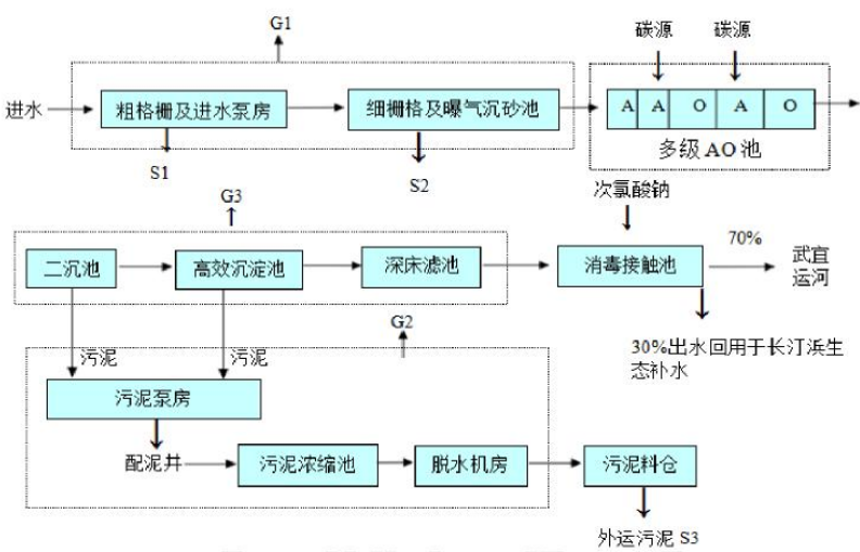
图 4-2 滨湖污水处理厂工艺流程图
