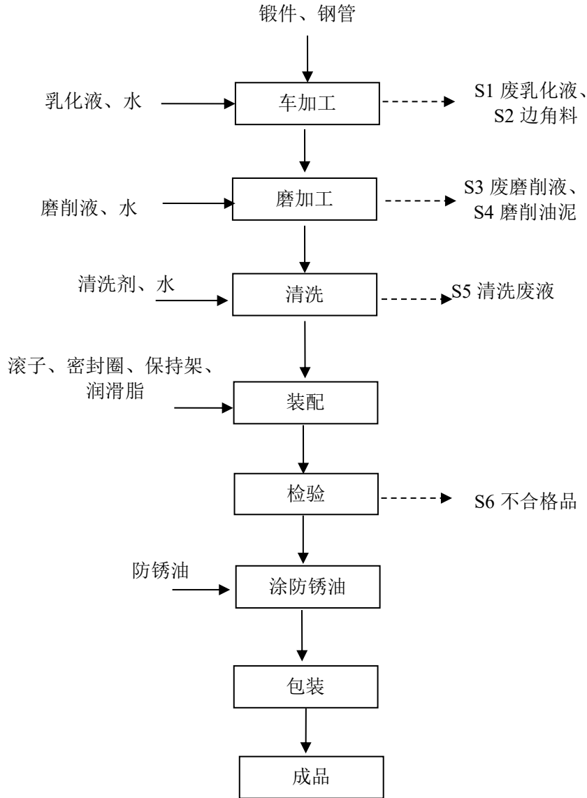
图 2-2 轴承生产工艺流程图
