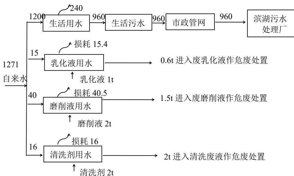
图 2-1 本项目水平衡图 (单位: t)
