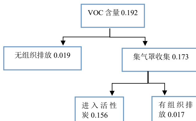
图2-3 本项目VOCs平衡图（单位：t/a）
