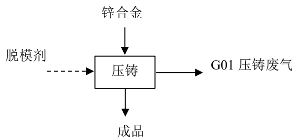
图 2-5 锌合金压铸件生产工艺流程图
