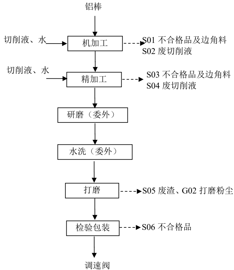
图 2-6 调速阀生产工艺流程图
