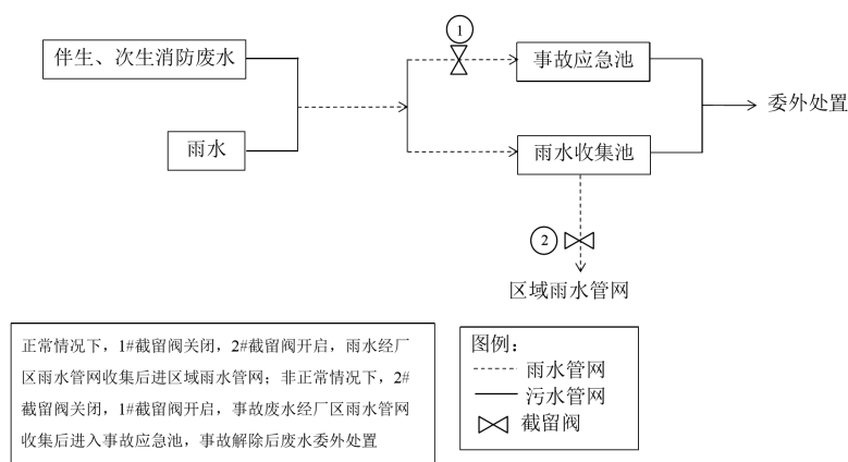
图 4-3 事故排水控制和封堵示意图
