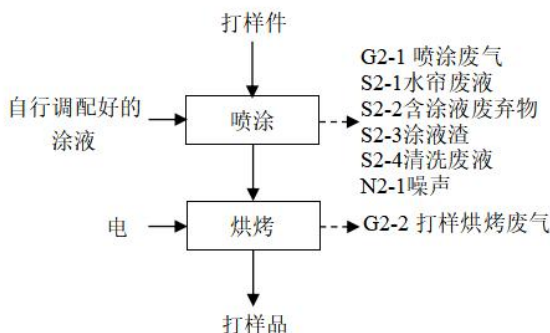
图 2-3 打样小试生产工艺流程图
