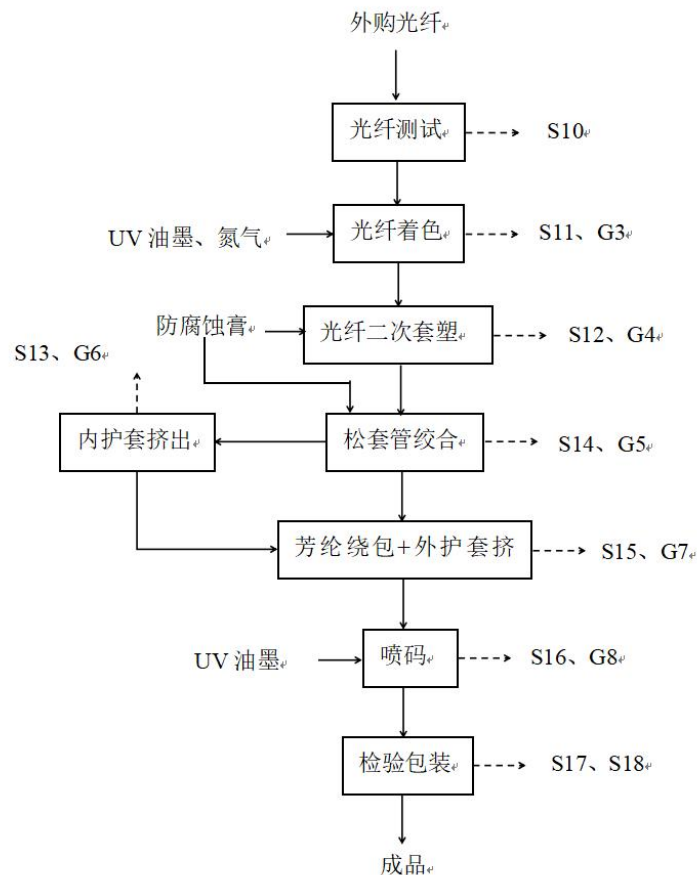
图 2.2-2 ADSS 光缆制造工艺流程及产污环节图
