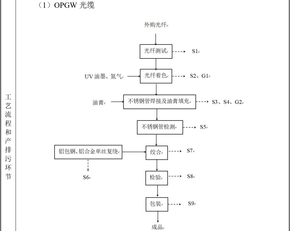
图 2.2-1 OPGW 光缆制造工艺流程及产污环节图
