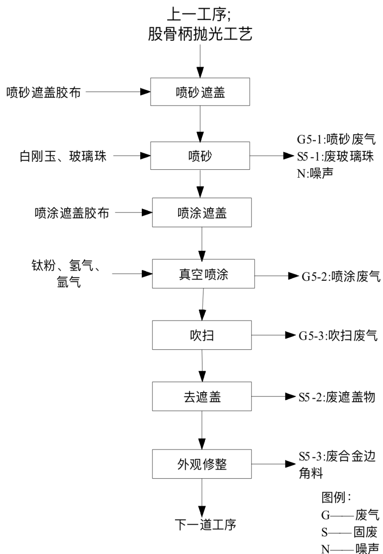
图 5 喷涂工艺
