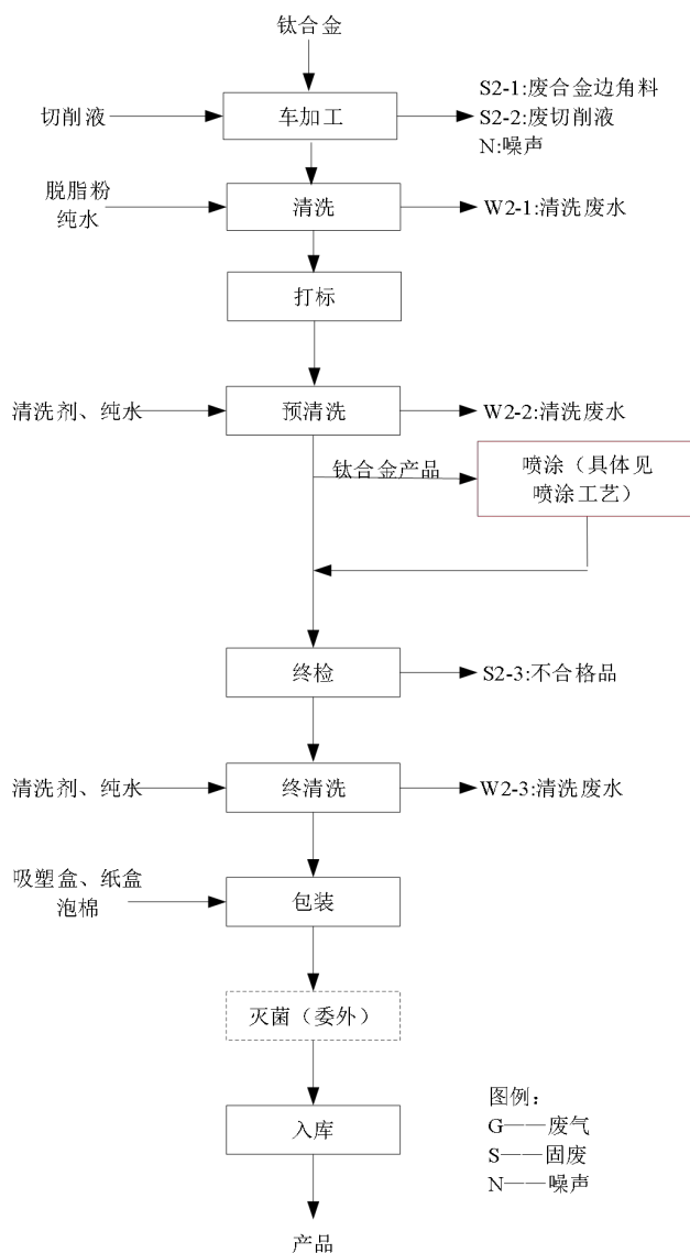
图 2-6 金属髌臼生产工艺流程图
