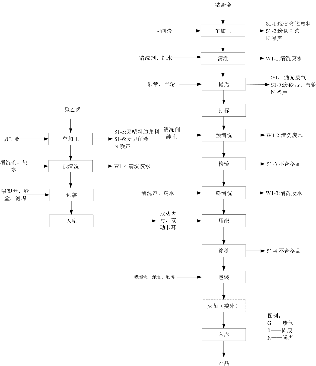
图 2-5 双动金属杯、金属球头生产工艺流程图
