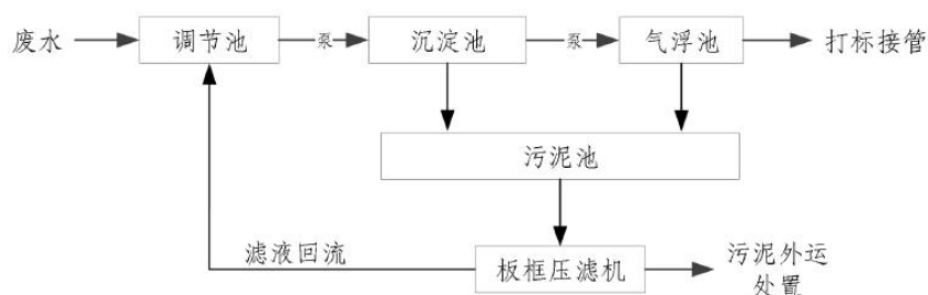
图 4-3 厂区现有污水处理工艺流程图
