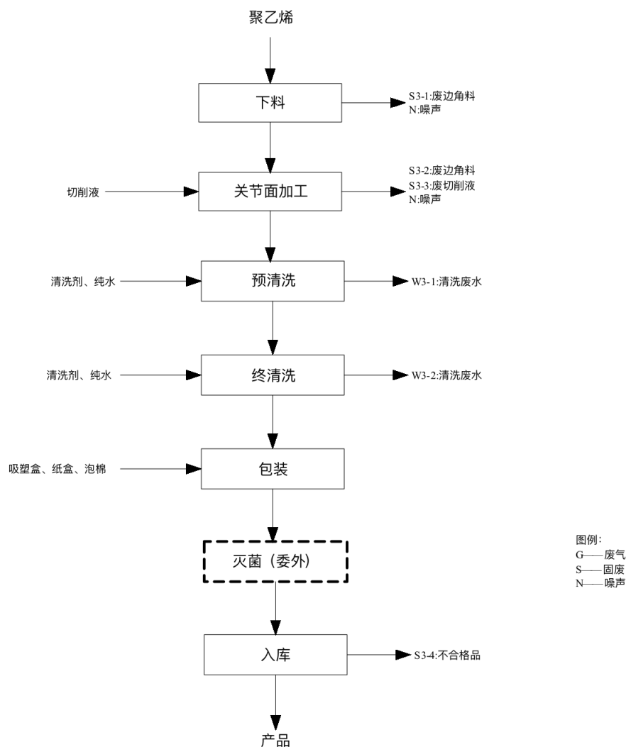
图 3 XPE 内衬生产工艺流程图
