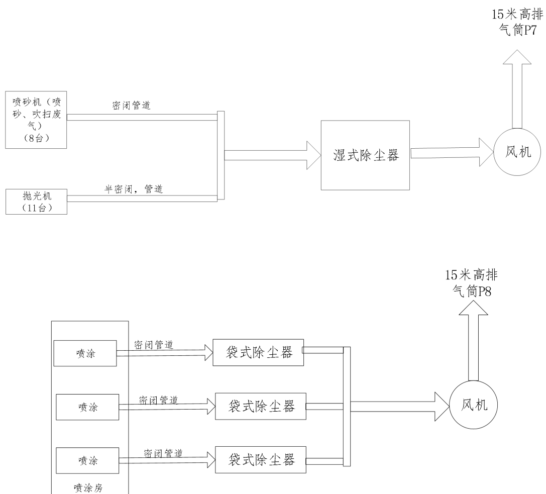
图 4-1 废气收集及处理工艺示意图
