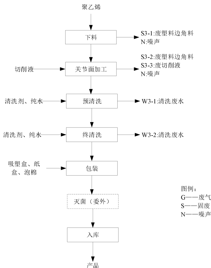
图 2-7 XPE 内衬生产工艺流程图
