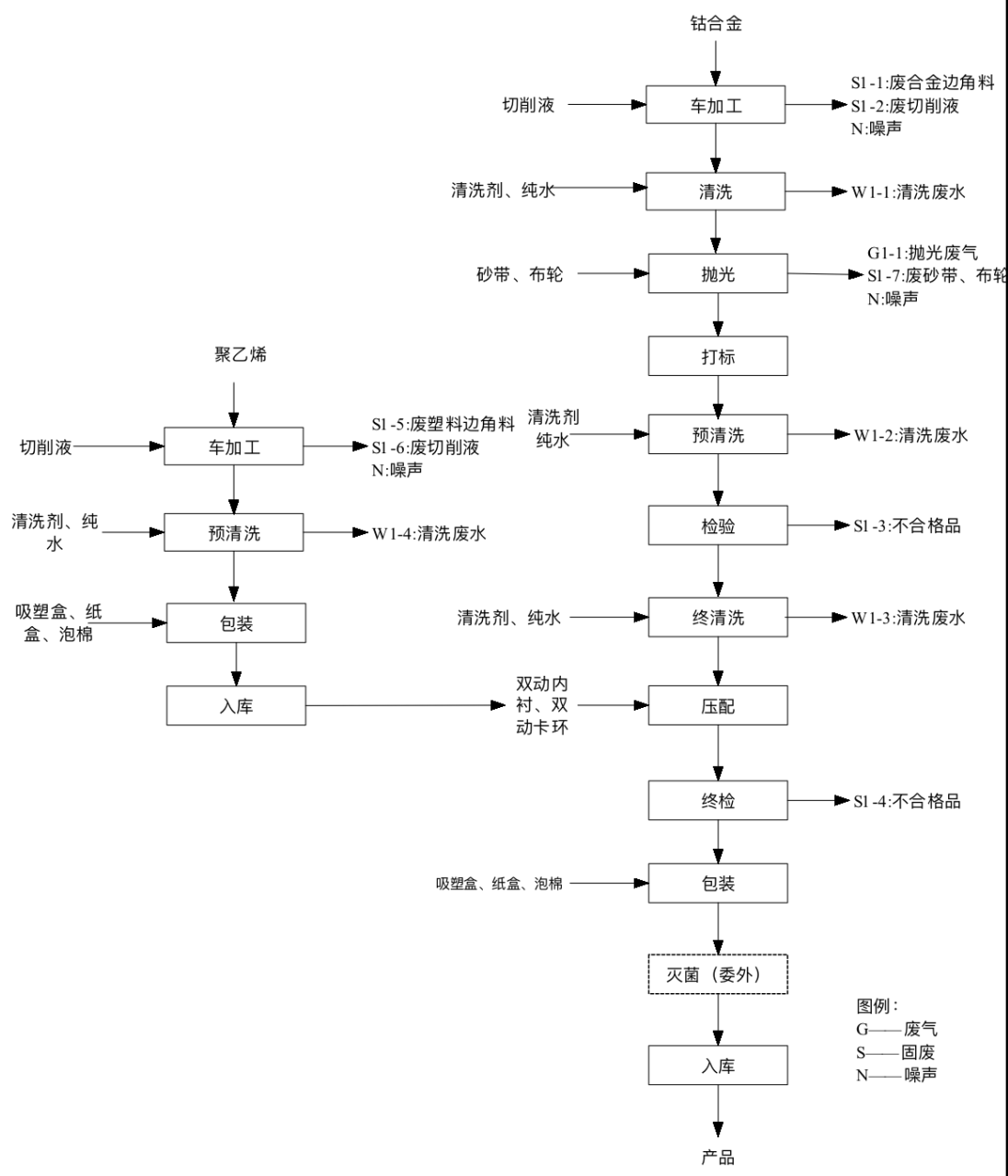
图 1 双动金属杯、金属球头生产工艺流程图
