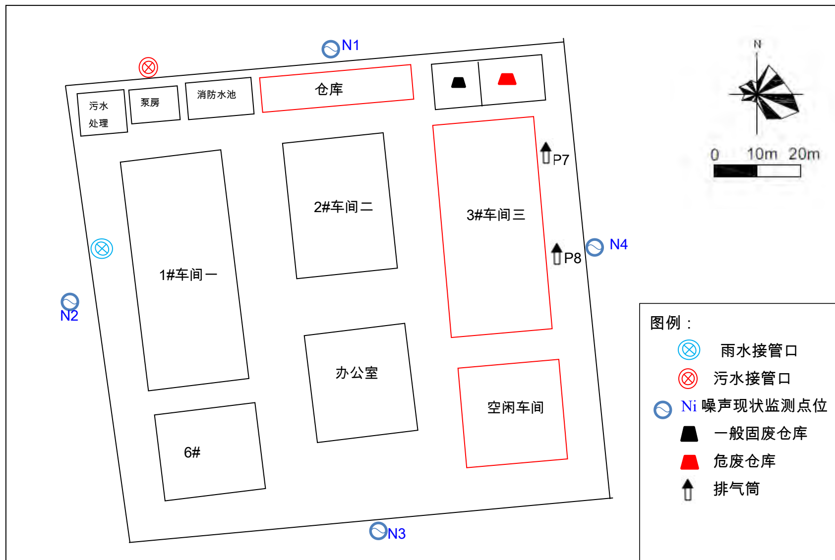
附图3-1 厂区平面布置图
