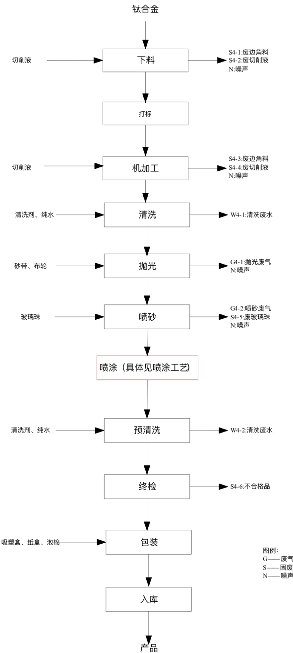
图 4 股骨柄生产工艺流程图
