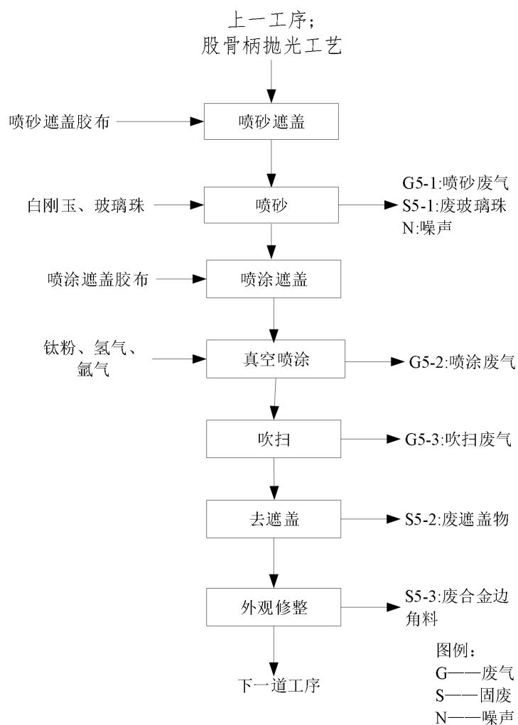
图 2-8 抛光后喷涂工艺
