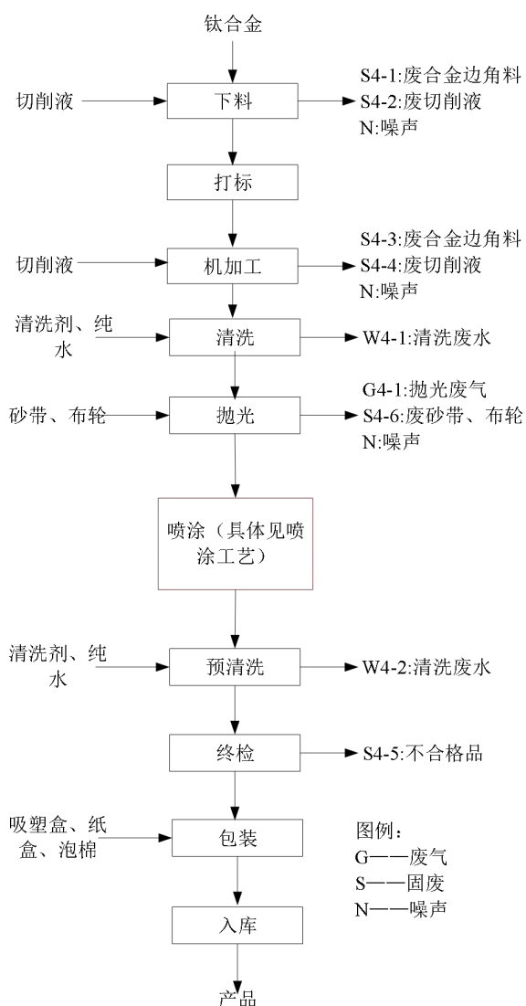
图 2-8 股骨柄生产工艺流程图
