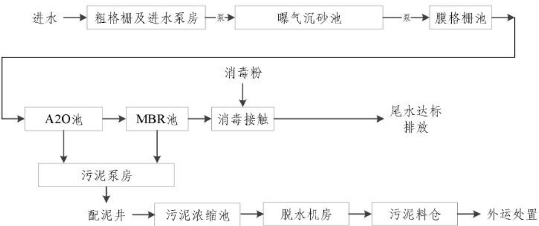
图 4-5 污水处理工艺流程图
