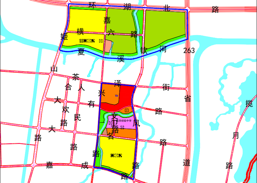
JZ0904、JZ0909基本控制单元部分地块
