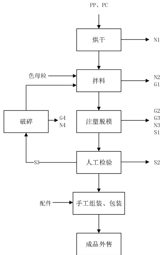
图 2-2 喇叭、蜂鸣器结构件及外壳生产工艺流程图 (注：Gn：废气污染物；Sn：固体废弃物；N：噪声)
