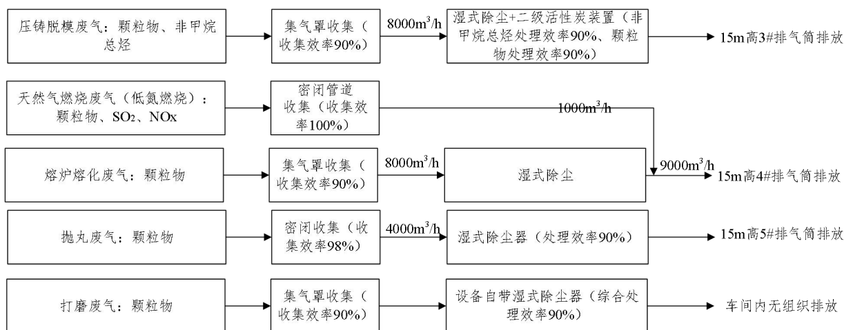
图 4-1 企业废气工艺示图
