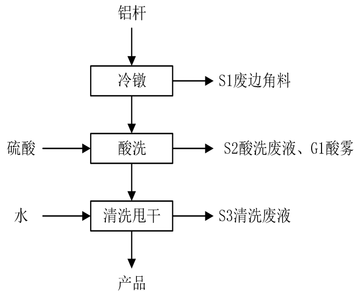
图 2-6 铆钉项目生产工艺流程图
