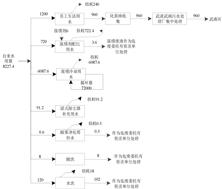
图 2-3 本项目建成后全厂水平衡图：t/a
