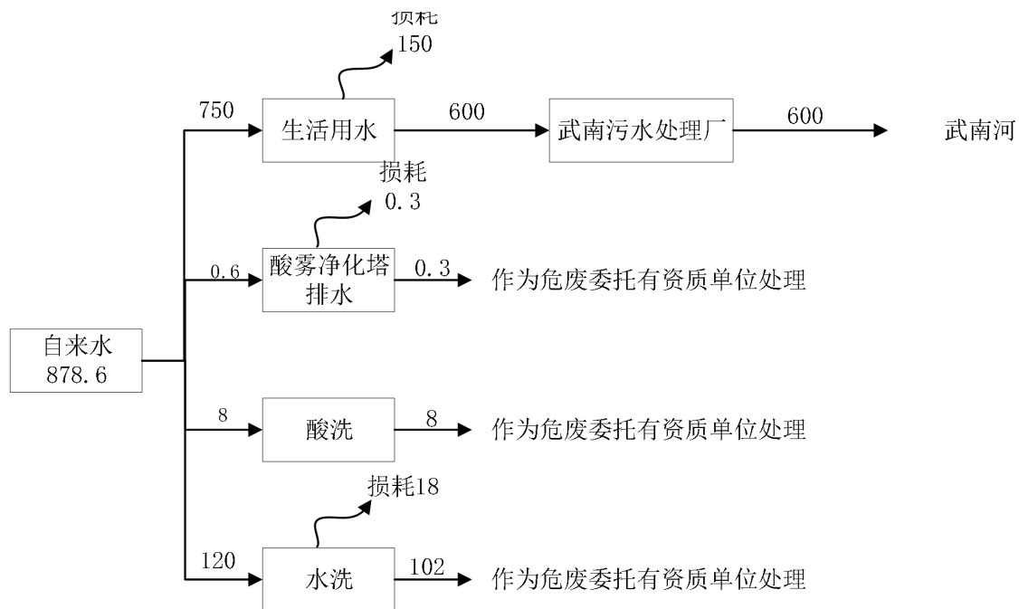
图 2-5 原有项目水平衡图：t/a
