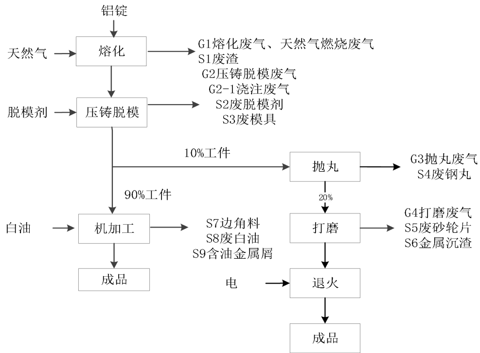
图 2-4 生产工艺流程图
