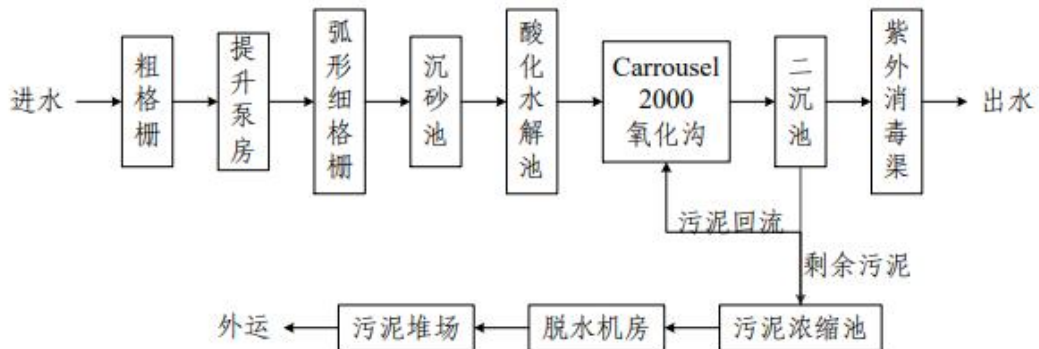
图4-2 武进武南污水处理厂污水处理工艺流程图
