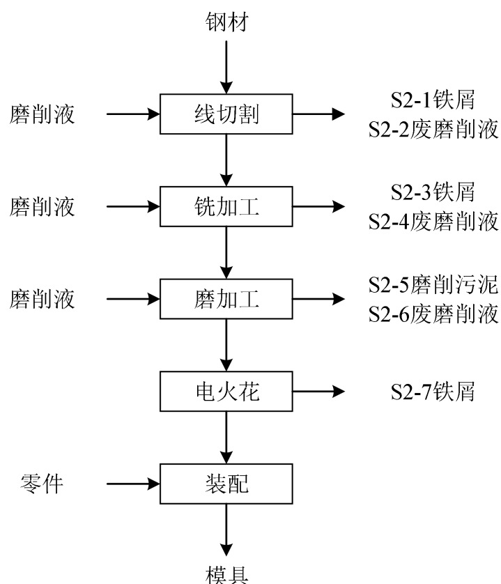
图 2-5 配套工艺流程图
