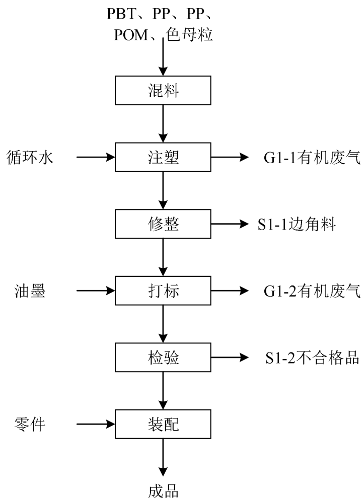
图 2-4 项目工艺流程图
