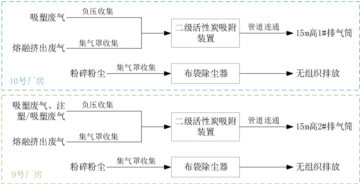
图 4-1 本项目废气收集治理方案示意图
