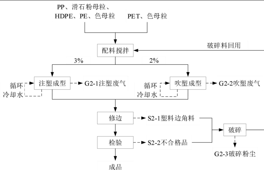
图 2-4 注塑件工艺流程图
