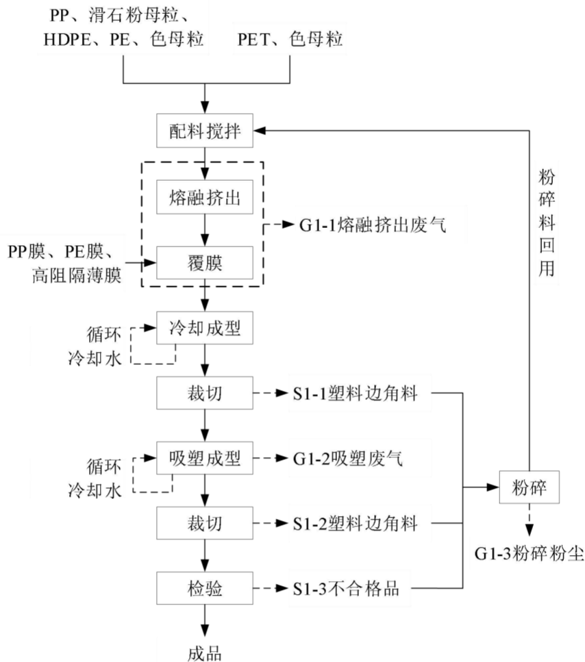
图 2-3 吸塑件生产工艺流程图
